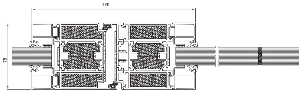
Ușă - vedere în secțiune
