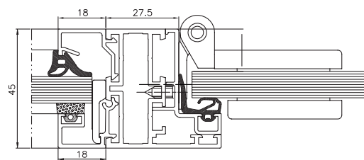
Montant de ușă – vedere în secțiune
