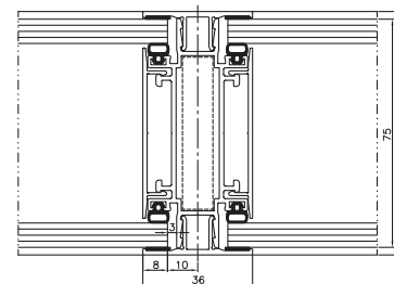
perete de 80 mm - vedere verticală
