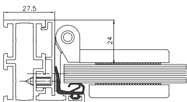
Ușă – vedere laterală
