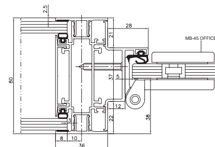
Ușă - vedere orizontală
