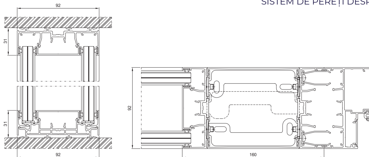
Perete despărțitor interior, secțiune transversală verticală Secțiune transversală orizontală prin montant și tocul ușii
