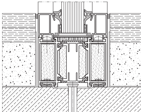
Perete vitrat îmbinat cu silicon – jos
