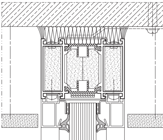
Perete vitrat îmbinat cu silicon – sus
