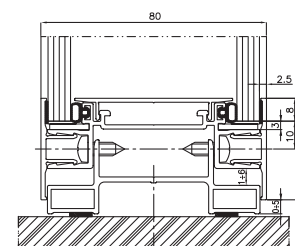
Traversă inferioară - vedere
