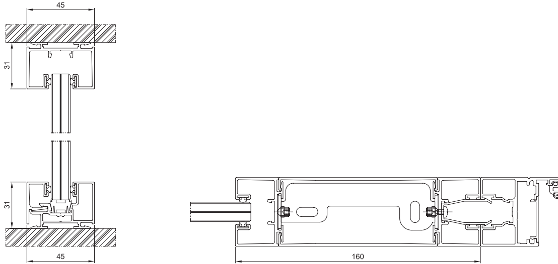
Perete despărțitor interior, secțiune transversală verticală Secțiune transversală orizontală prin montant și tocul ușii
