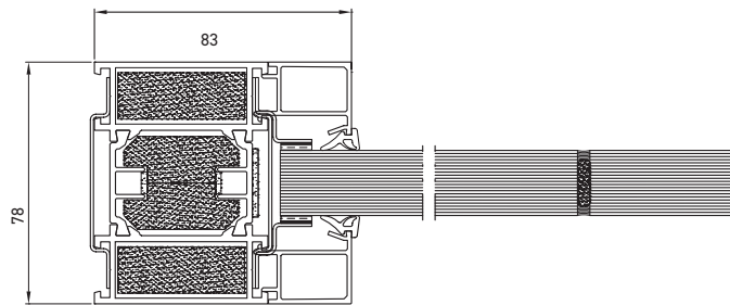
Toc de perete fix - vedere în secțiune
