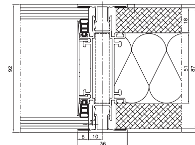
perete de 92 mm - vedere verticală
