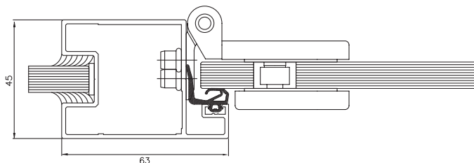
Montant de ușă și traversă superioară – vedere
