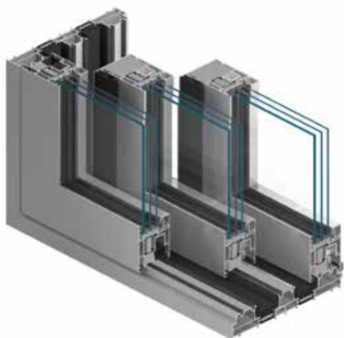
ramă cu 3 șine
